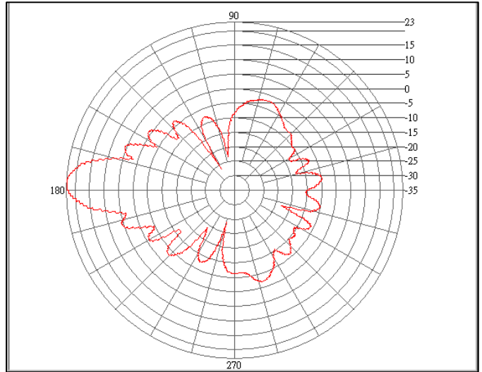
E-Plane
