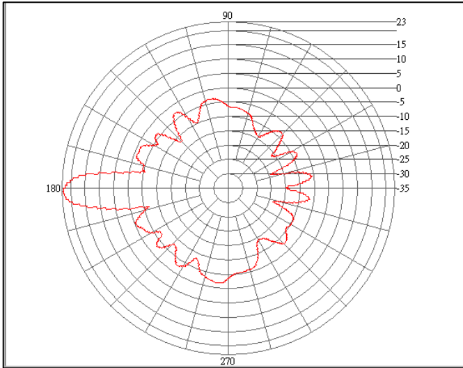
H-Plane
